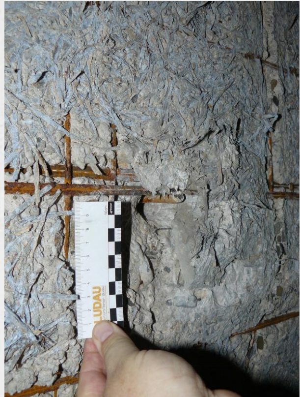
BETONINSTANDSETZUNG
