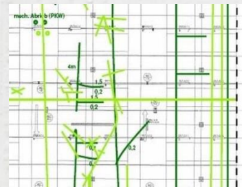
Beispielhafte Rissaufnahme und Rissfortschreibung über mehrere Inspektionstermine
