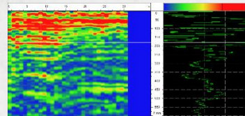
Schulung über Möglichkeiten und Grenzen der zerstörungsfreien Messtechnik, Beispiel Ultraschallmessung
