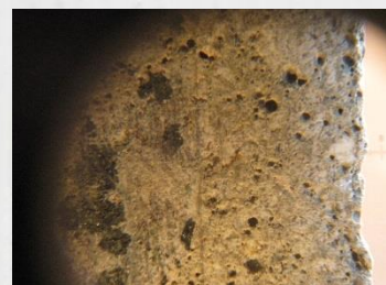
LP-Beton unter dem Lichtmikroskop bei 10facher Vergrößerung
